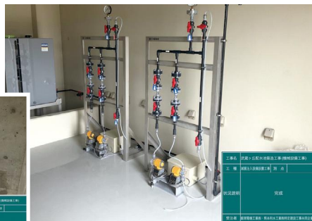
滅菌注入設備設置状況
