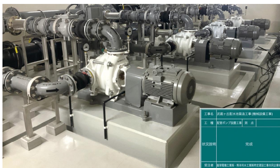
配水ポンプ・配管 設置状況
